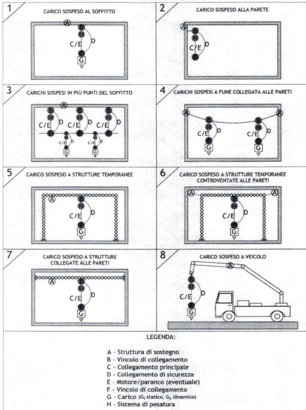
Fig. 1 - Schemi ricorrenti di tipologie di carichi sospesi
